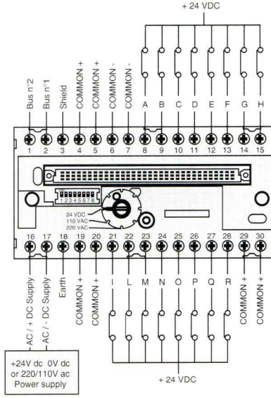
Type/Unit : ICSO 08 R1 Binary output module
