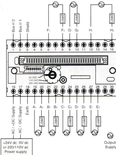
Type/Unit : ICSO 08 R1 Binary output module
