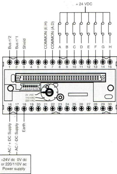
Type/Unit : ICSI 08 E3/E4 Binary input module
