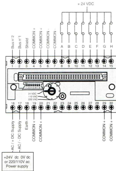
Type/Unit : ICSI 08 D1 Binary input module
